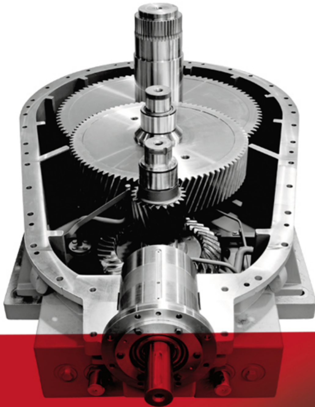
Mühlengetriebe
